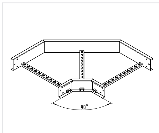
90° Bend KTCL 50 / 100 / 130 . B / Width / 90°
