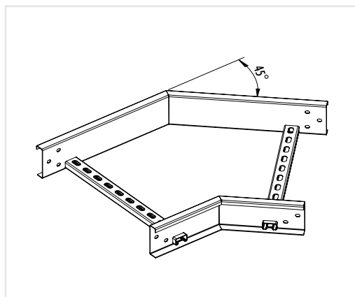
45° Bend KTCL 50 / 100 / 130 . B / Width / 45°
