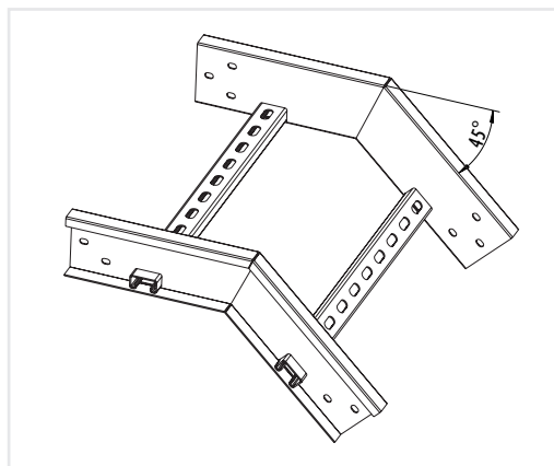
45° External Riser KTCL 50 / 100 / 130 . ER / Width / 45°
