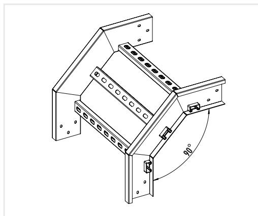
90° External Riser KTCL 50 / 100 / 130 . ER / Width / 90°
