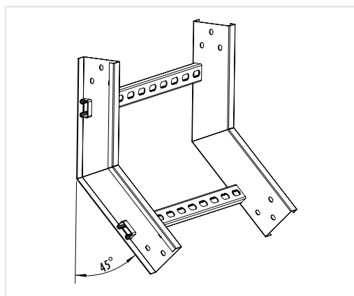
45° Internal Riser KTCL 50 / 100 / 130 . IR / Width / 45°
