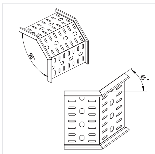
90 Deg / 45 Deg External Riser 90度/45度外曲
