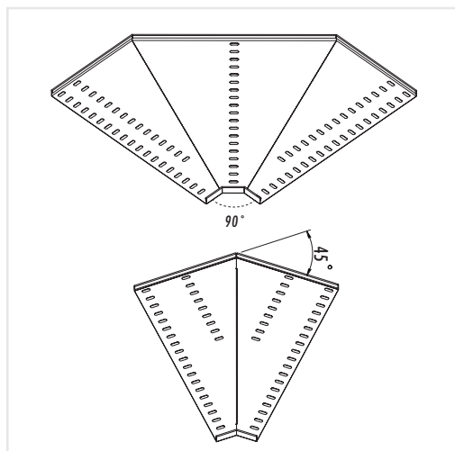
90 Deg / 45 Deg Bends 90度/45度大面曲
