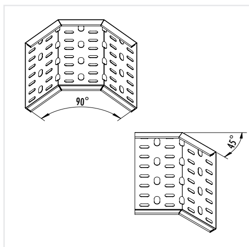
90 Deg / 45 Deg Internal Riser 90度/45度內曲
