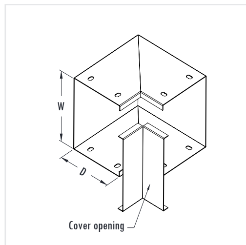
90 degree Internal Opening Elbow (90度 直角內曲)
