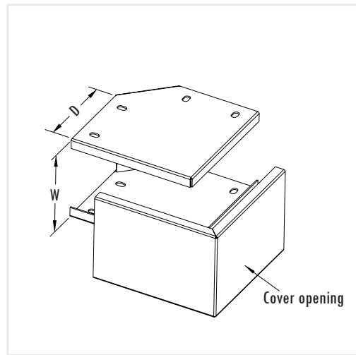
90 degree External Opening Bend (90度 外曲)
