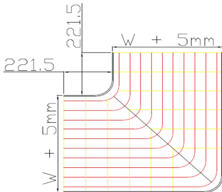
CABLE BASKET 90DEG DEG. BEND
