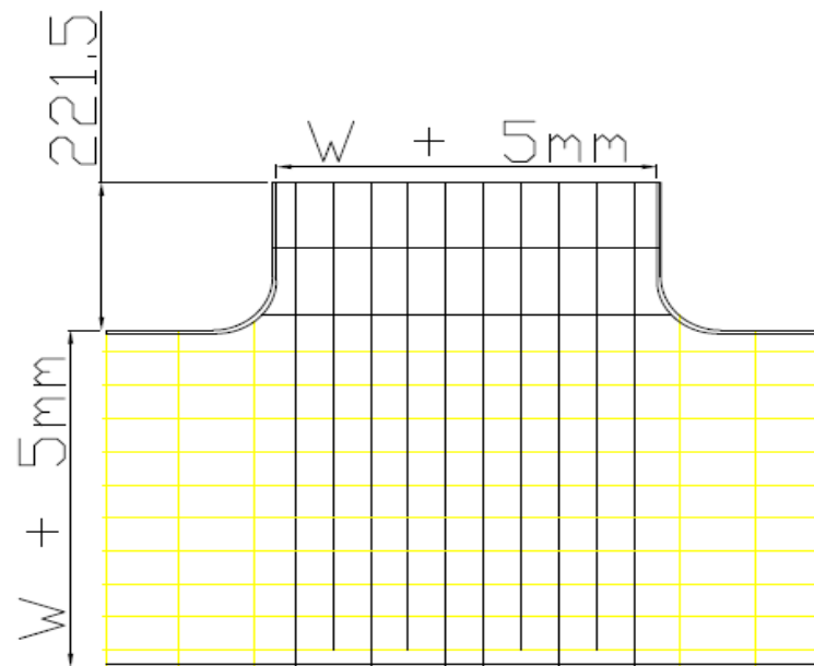
CABLE BASKET TEE
